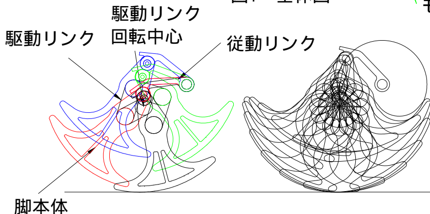
図2 脚の構造及び軌跡
