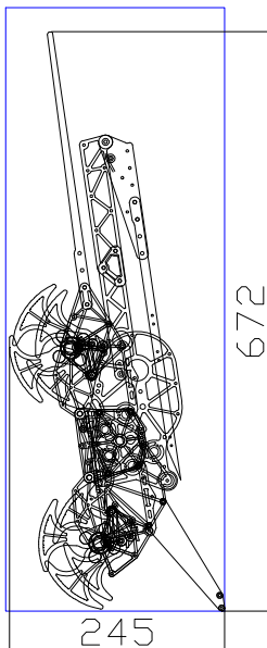
図5 スタート時の姿勢
