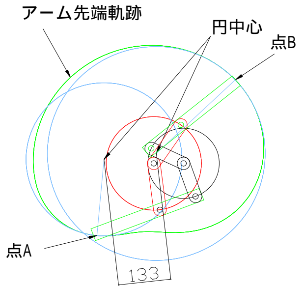
図4 アームの先端軌跡
