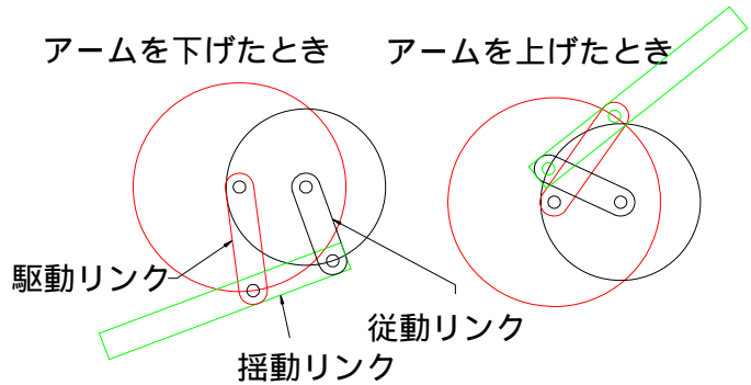
図3 アームの構造
