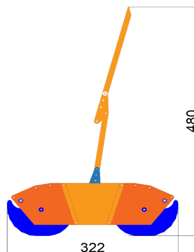
図2. スタート時の姿勢及び寸法[mm]
