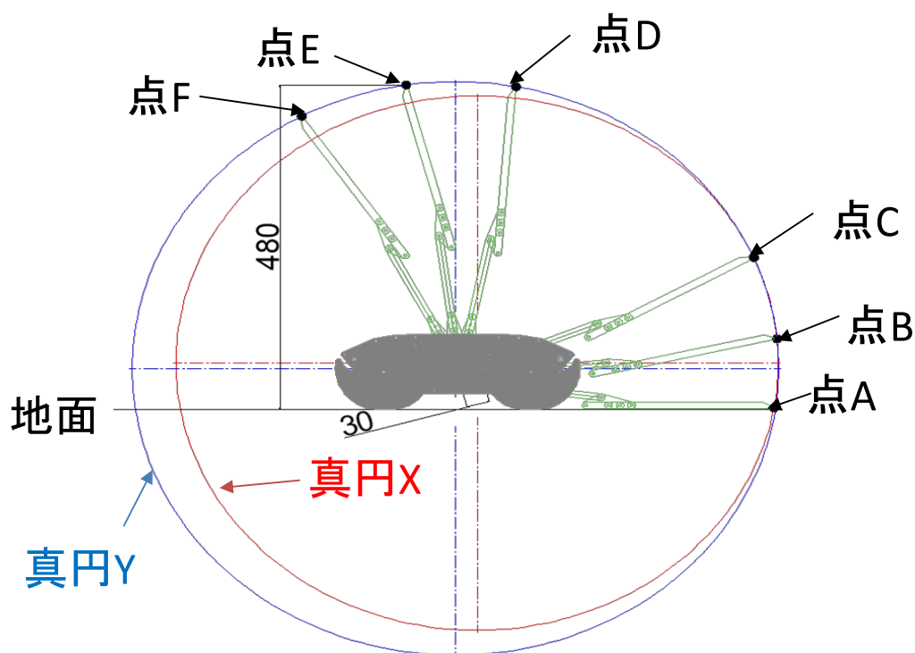
図6. アーム軌跡[mm]
