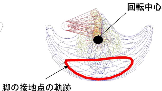
図4. 脚の軌跡
