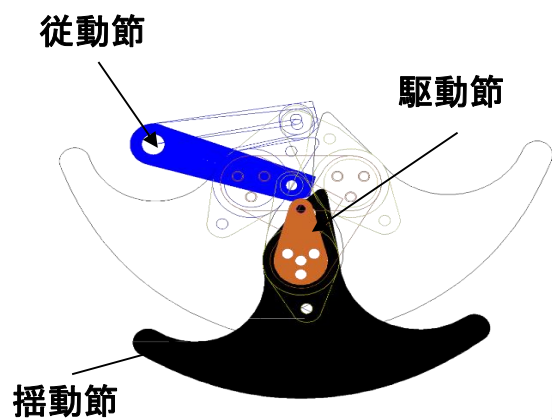
図3. 脚の機構
