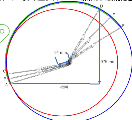
図6 アーム機構軌跡図
