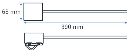
図8 第二アーム換装図
