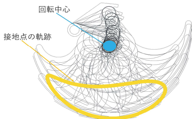
図4 脚機構の軌跡
