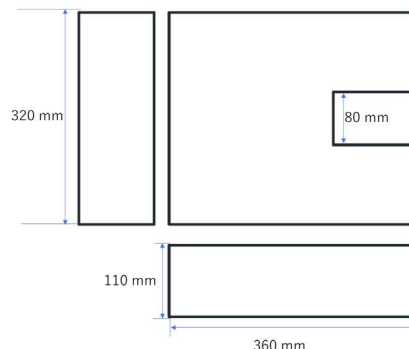
図10 機体側面換装図
