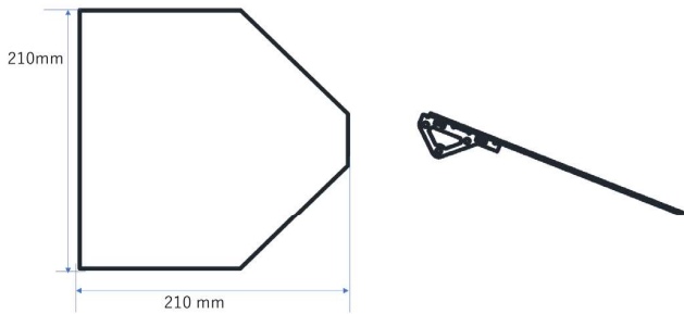
図7 シールド換装図
