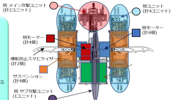
図3：部品レイアウト (スタート後姿勢 平面図)
