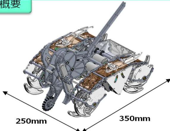
図1：スタート前姿勢 全体図
