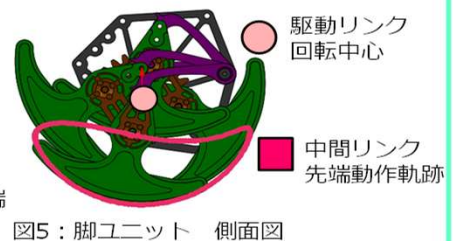
図5：脚ユニット 側面図
