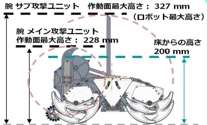
図2：スタート前姿勢 側面図
