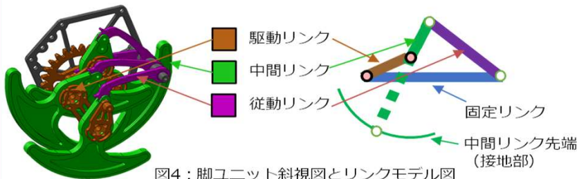
図4：脚ユニット斜視図とリンクモデル図
