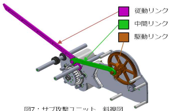
図7: サブ攻撃ユニット 斜視図
