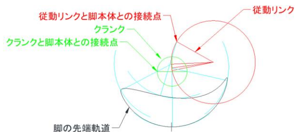
図4 脚の軌跡
