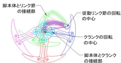
図3 脚の構造
