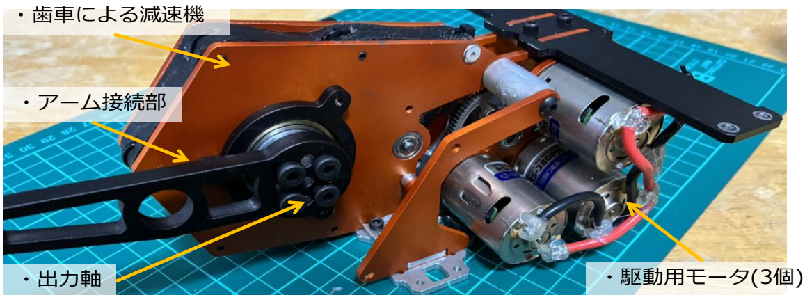
アームユニット（構造説明のため機構部のみの図）
