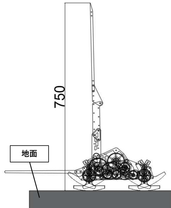
図5 地面からのアーム振り上げ高(mm)
