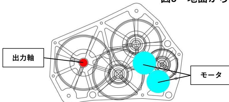
図6 アーム機構のモータ及び出力軸
