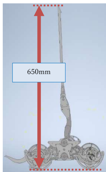
図8：スタート後 アーム作動最大高さ
