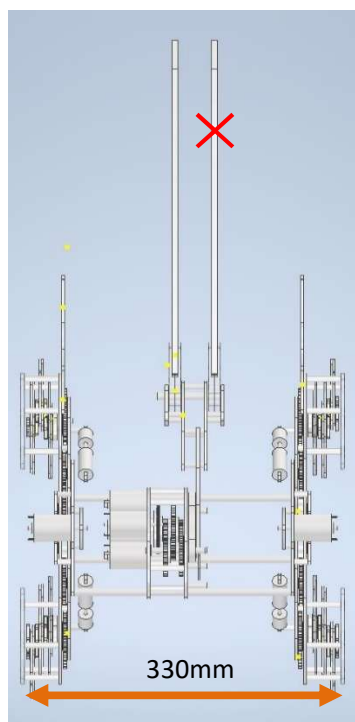
図6：スタート姿勢 （背面図）
