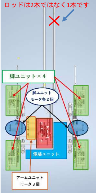
図1：ユニット配置図 (上面図)
