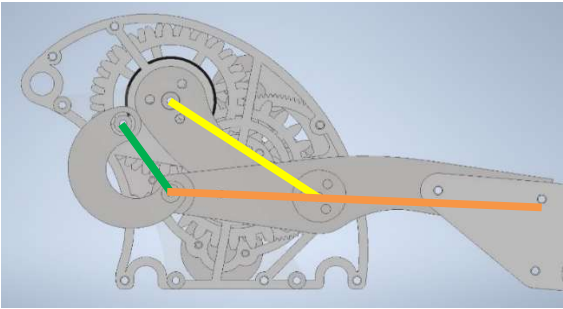
図4：アームの概要
