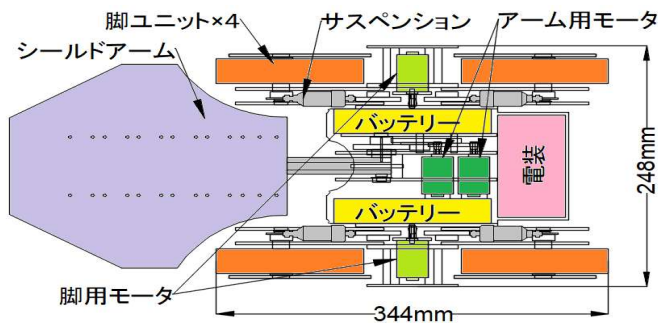
機体概要
