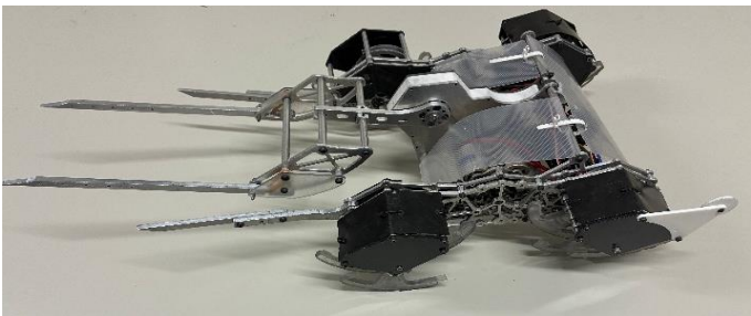
【図2】全体図(展開後)
