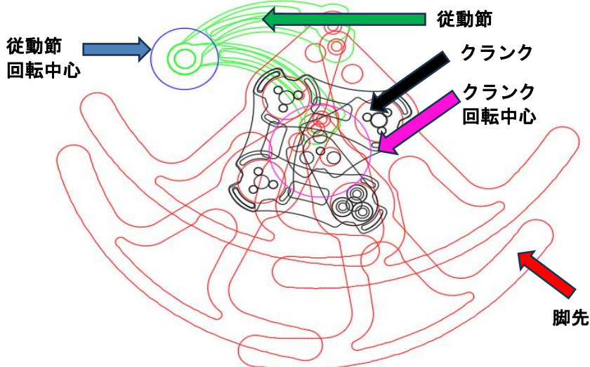
【図4】 脚の機構
