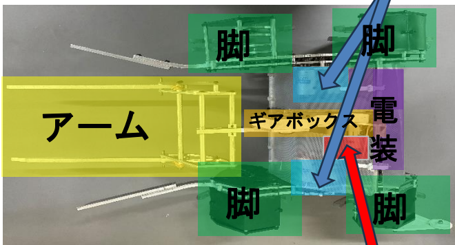
【図3】配置図
