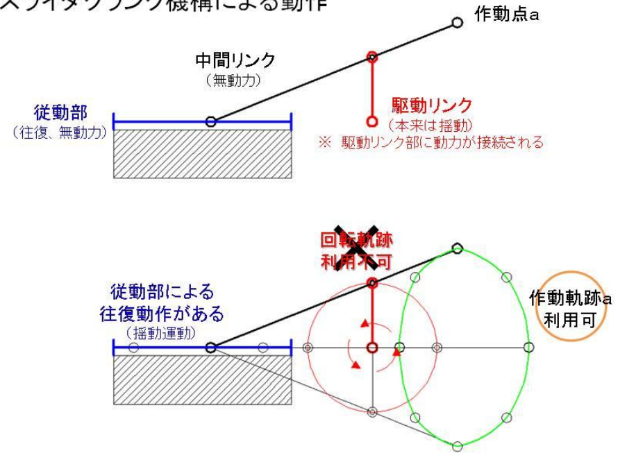
揺動リンク機構 参考例 スライダリンク機構による動作
