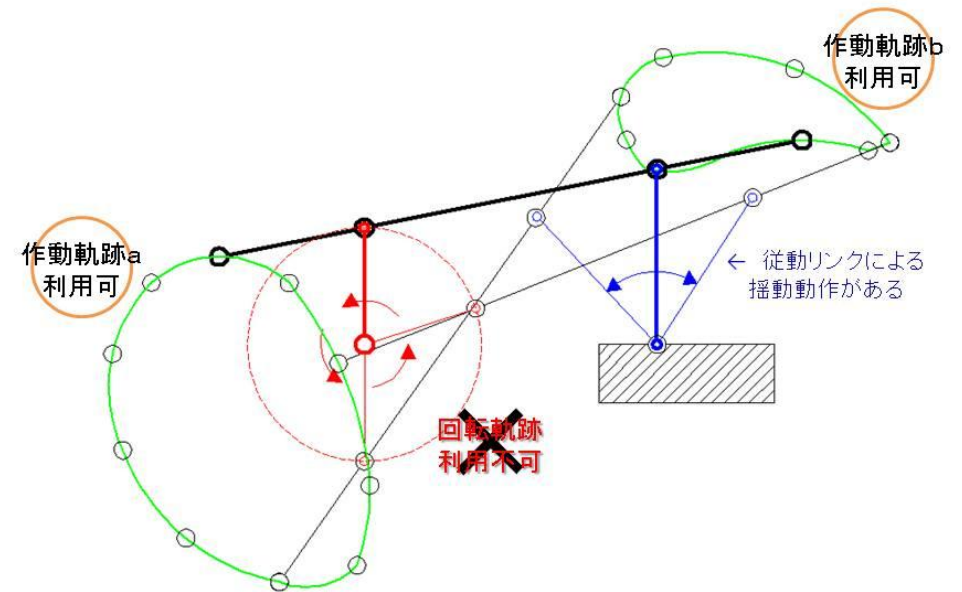
揺動リンク機構 参考例: 四節リンク機構による動作軌跡
